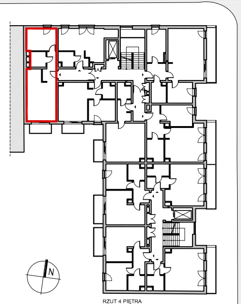
RZUT 4 PIĘTRA
